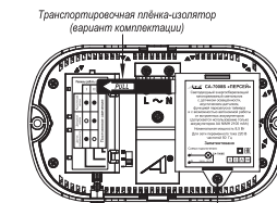
Рисунок 4. Светильника CA-7008Б. Вид сзади
